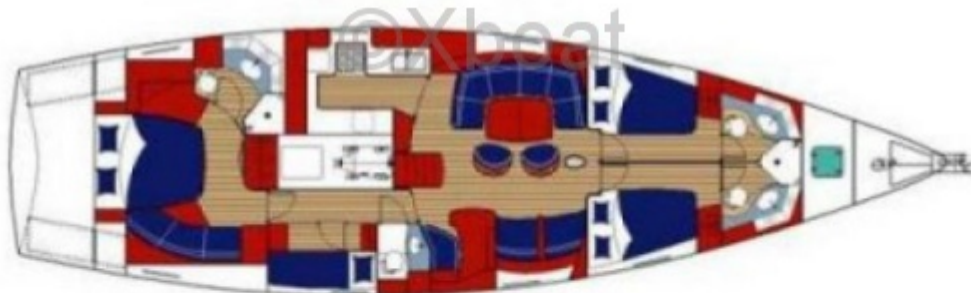
Version 1 cabine propriétaire arrière - 1 cabine coursive - 2 cabines avant 1 owner aft cabin - 1 watch cabin - 2 forward cabins version
